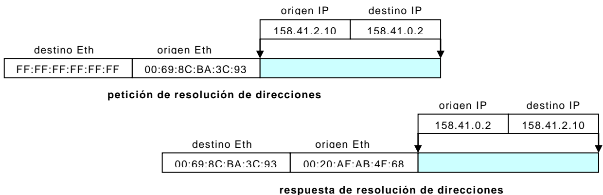
Fig. 12 - Intercambio de mensajes
