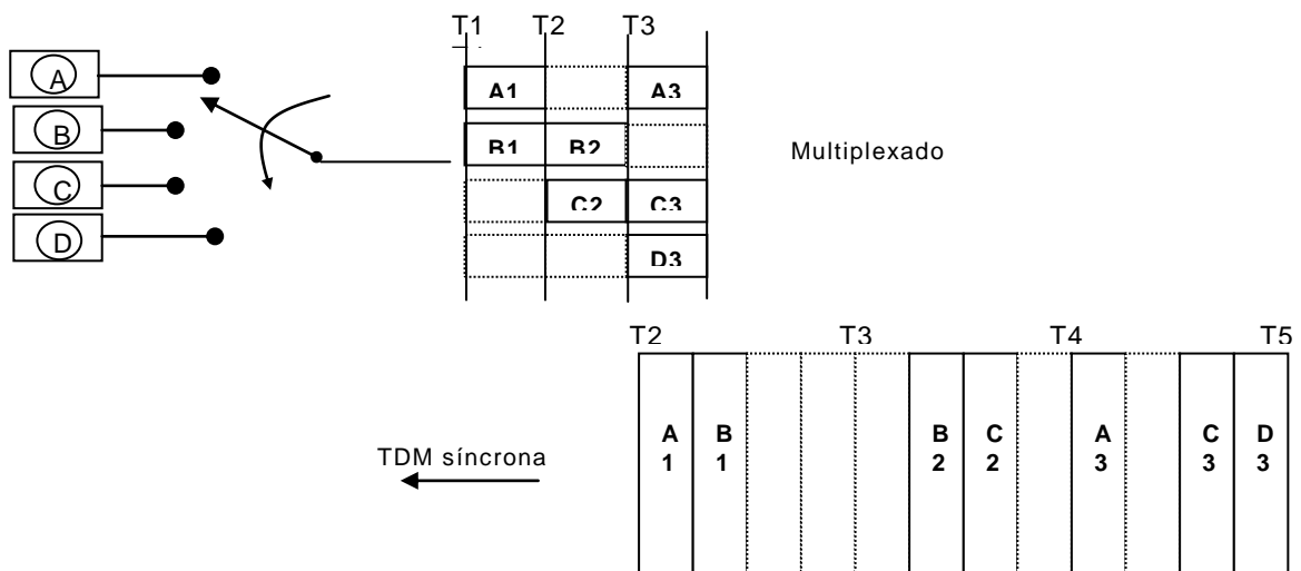
Fig. 22 - Multiplexado síncrono
