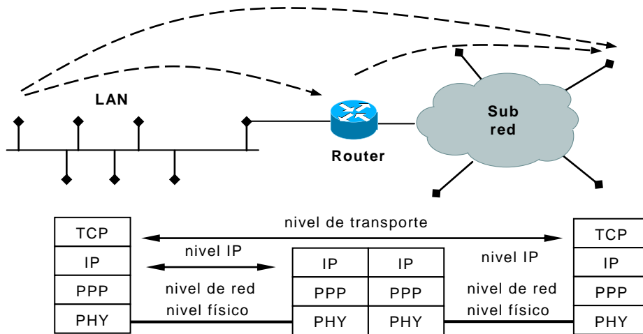
Fig. 6 - Arquitectura de protocolos en una internet IP
