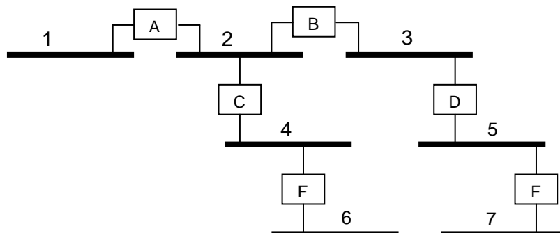
Fig. 21 - Ejemplo de Spanning Tree
