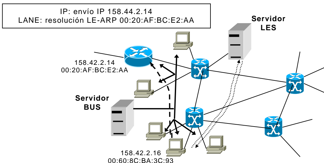
Fig. 48 - Funcionamiento IP sobre LANE (paso 2)
