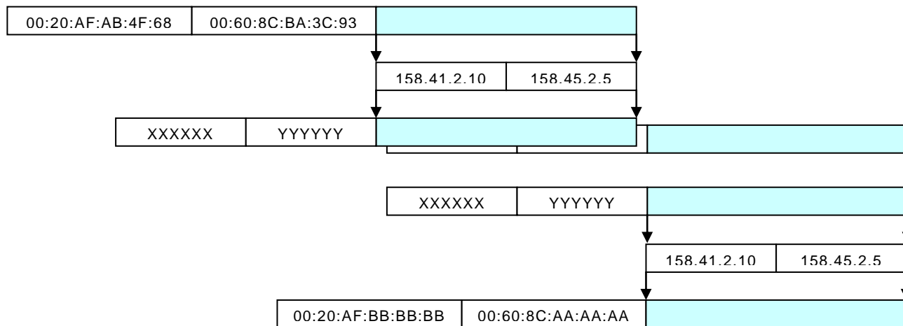
Fig. 16 - Encapsularlo IP en la trama de la subred 158.44.0.0
