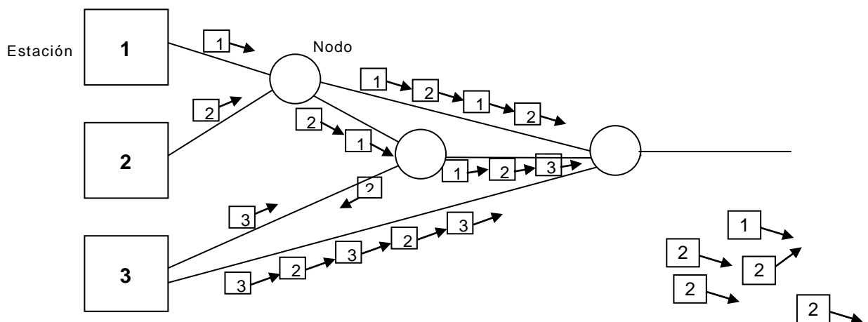
Fig. 25 - Encaminamiento en modo datagrama
