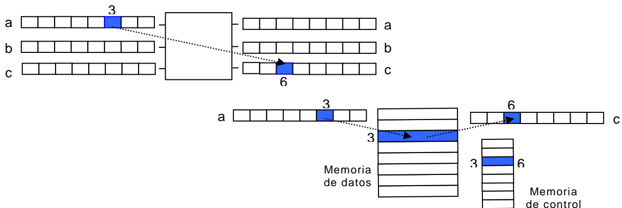
Fig. 23 - Conmutador de circuitos
