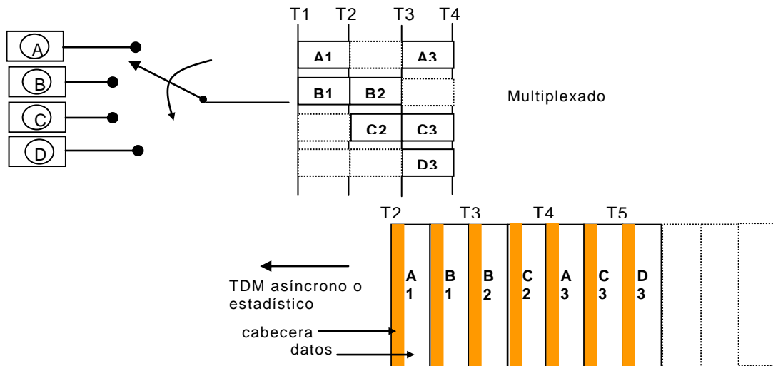
Fig. 24 - Multiplexado asíncrono
