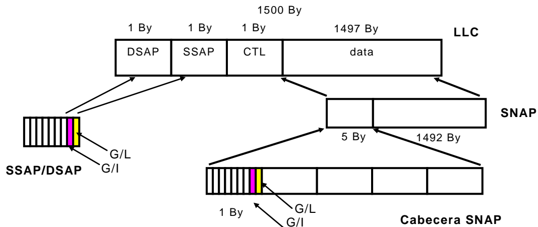
Fig. 9 - Encapsulado LLC/SNAP
